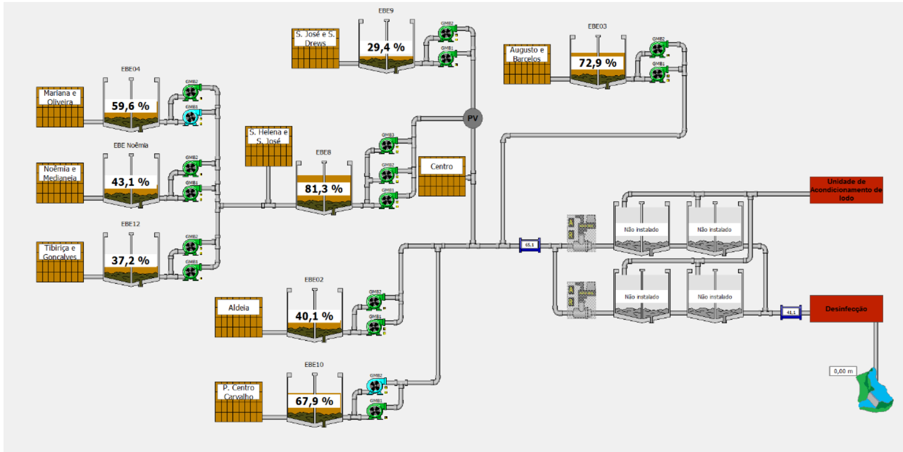
Figura 21 – Fluxograma do SES.
