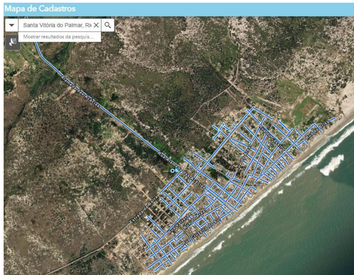
Figura 22 – adutoras e redes de distribuição de água (Praia do Hermenegildo).
