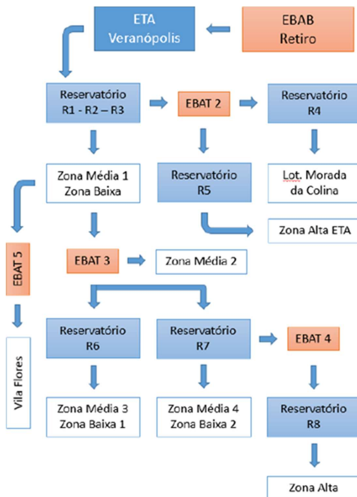
Figura 18 – Fluxograma do SAA (1/2).
