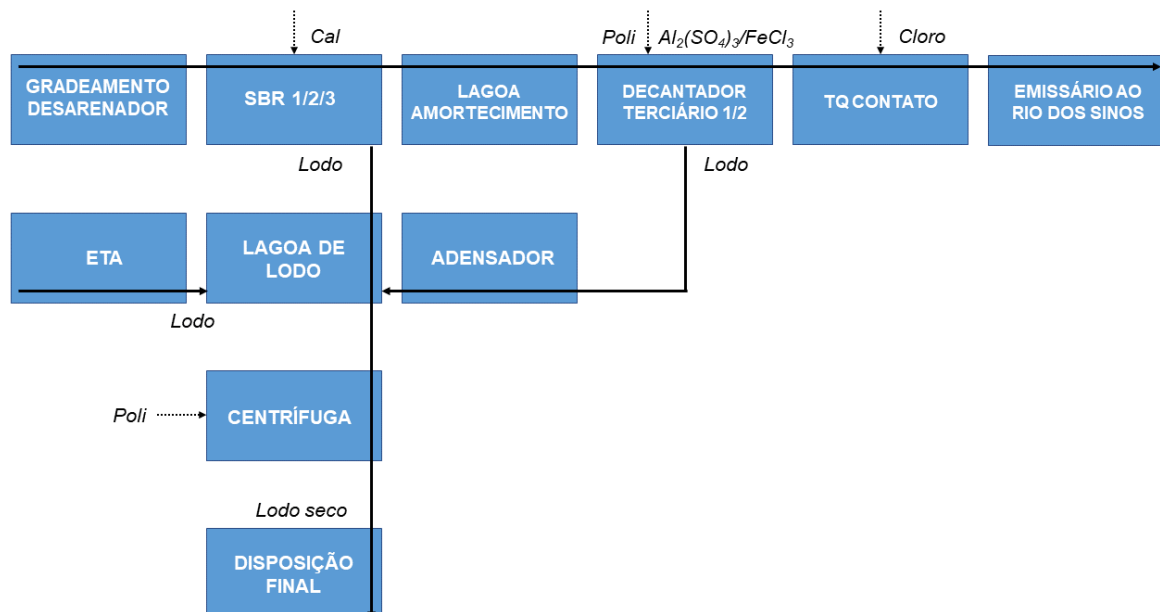
Figura 120 – Fluxograma da ETE componente do SES Esteio-Sapucaia do Sul.
