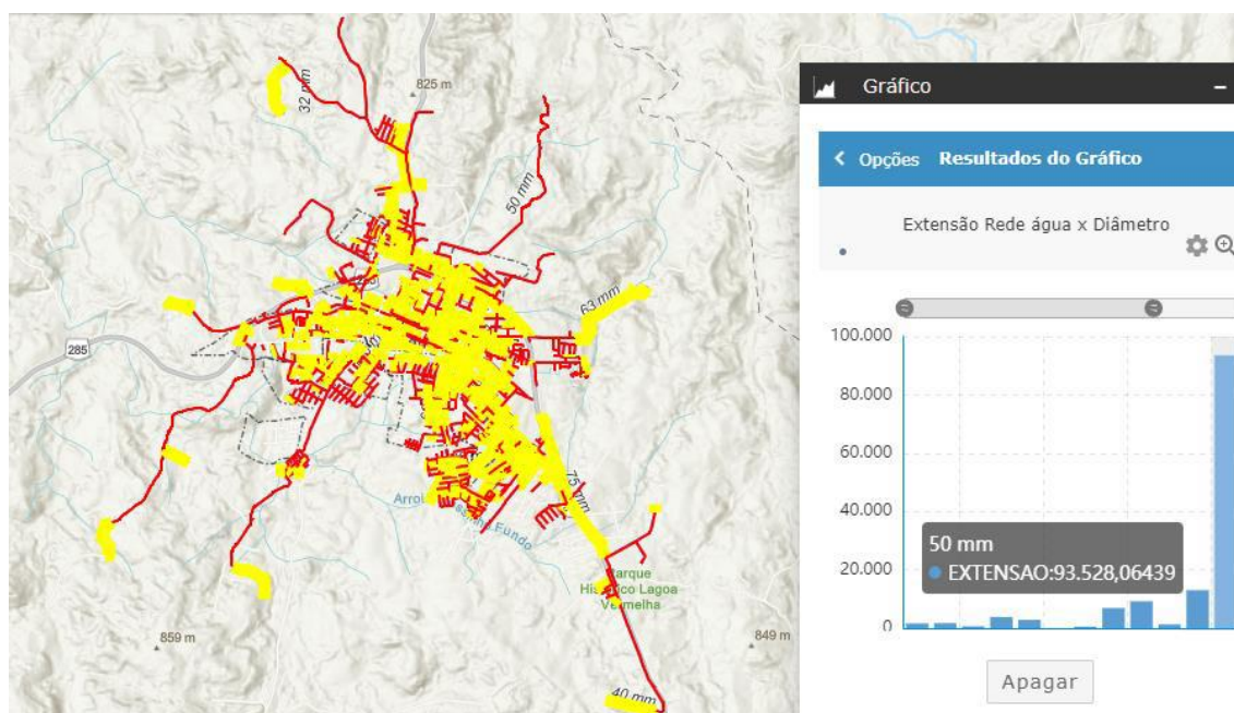
Figura 20 – Extensão rede água vs. diâmetro.
