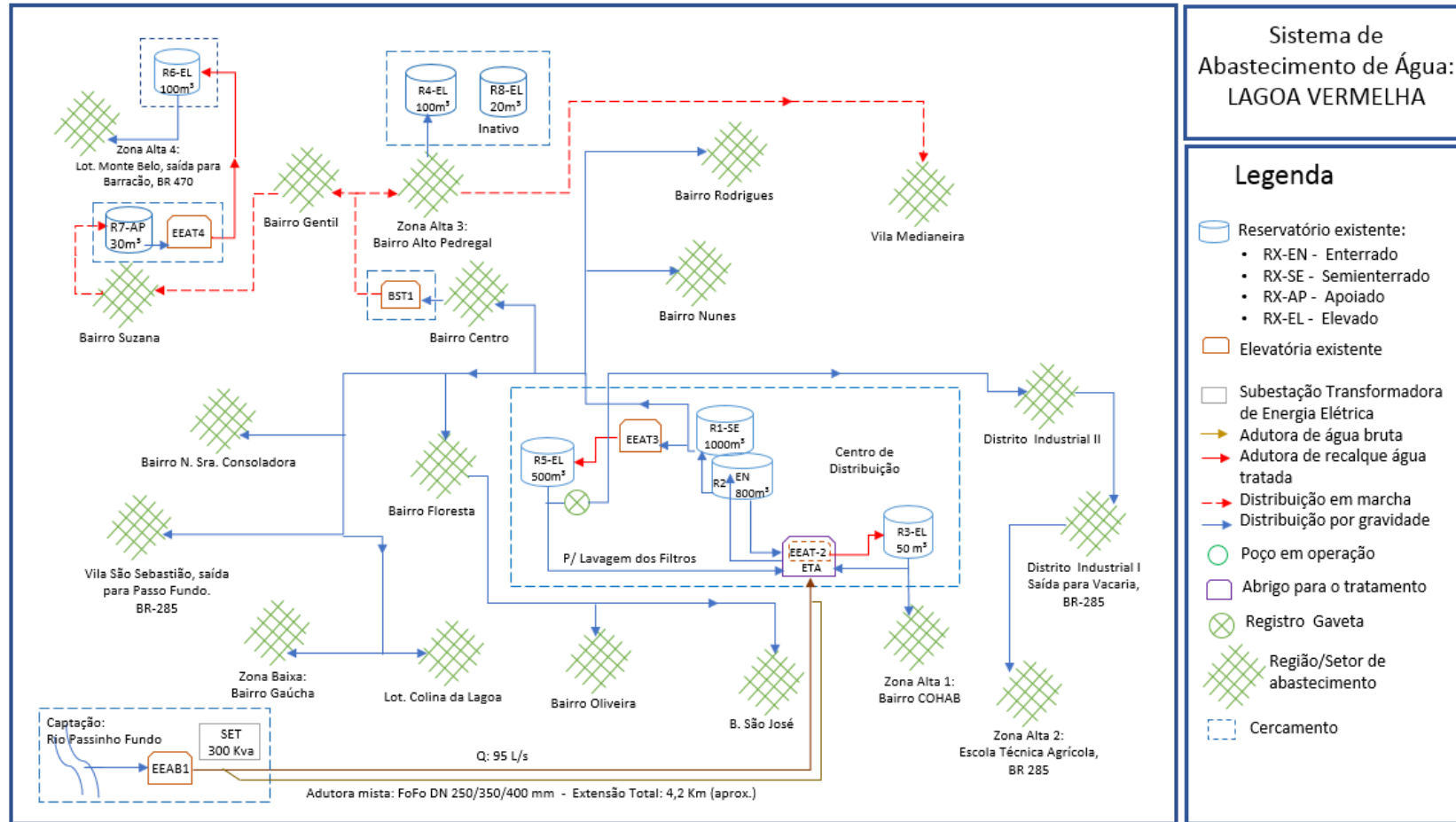
Figura 21 – Fluxograma do SAA.
