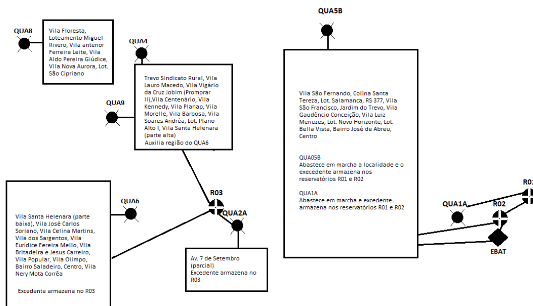
Figura 19 – Croqui da distribuição de água no município de Quaraí.
