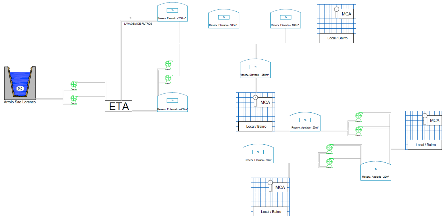
Figura 23 – Fluxograma do SAA.
