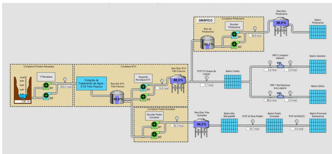
Figura 21 – Fluxograma do SAA.
